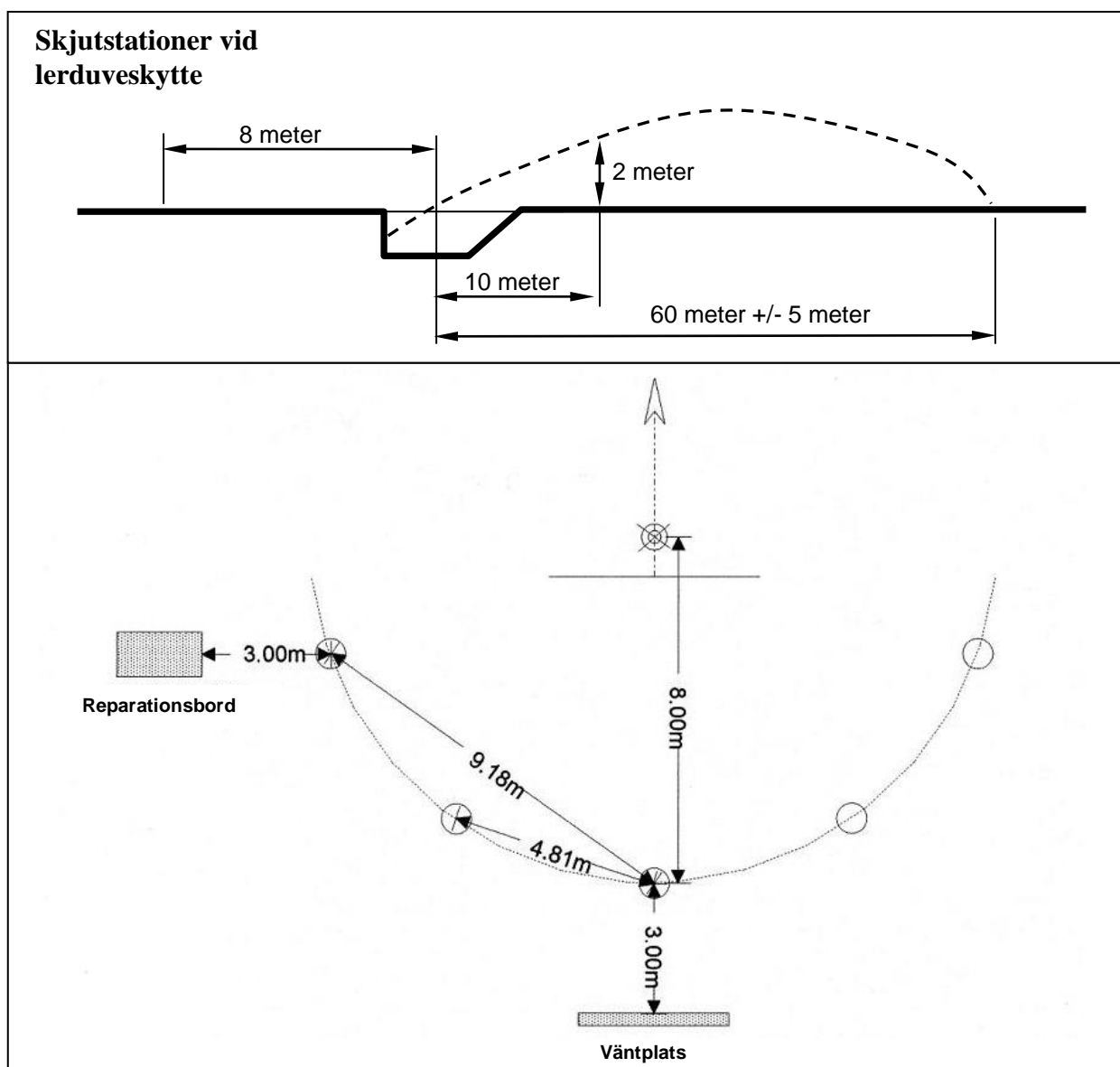
Figur 1. Skjutstationens utformning.
